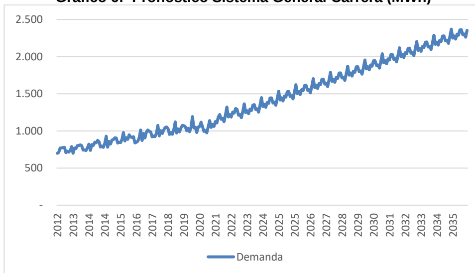
Gráfico 6: Pronóstico Sistema General Carrera (MWh)
