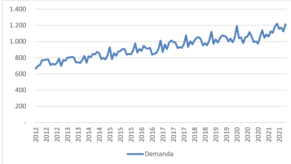
Gráfico 2: Demanda mensual de energía en el sistema General Carrera (MWh)
