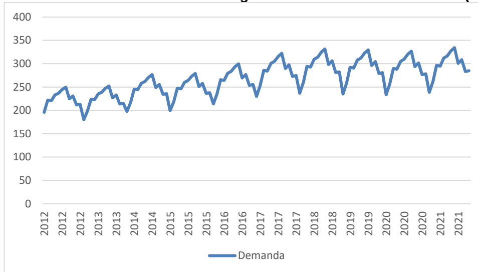
Gráfico 4: Demanda mensual de energía en el sistema Puerto Cisnes (MWh)
