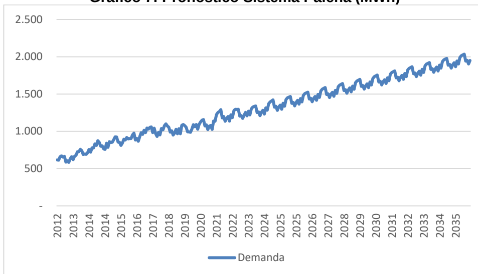
Gráfico 7: Pronóstico Sistema Palena (MWh)
