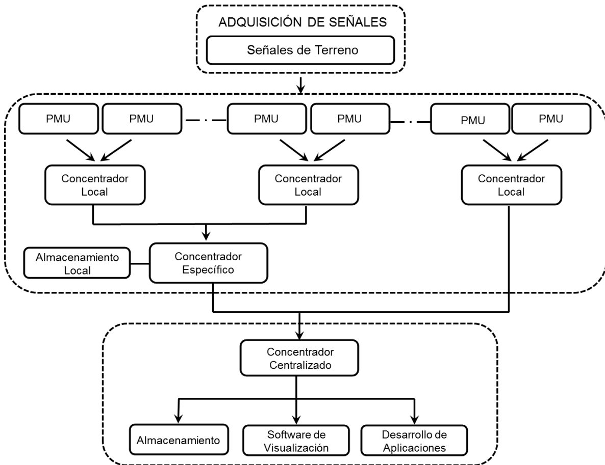
Figura 5: Arquitectura distribuida para el módulo de medición fasorial
