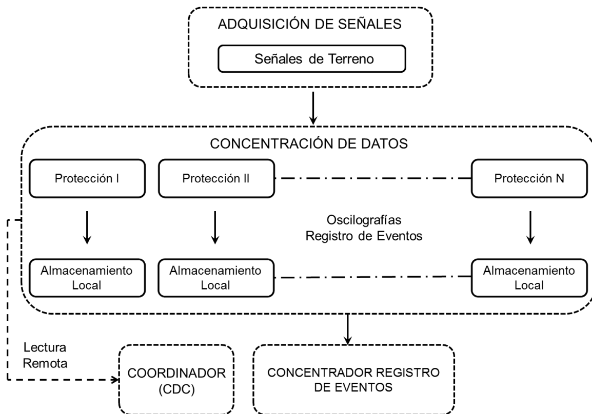
Figura 3: Arquitectura del módulo para registro de protecciones eléctricas
