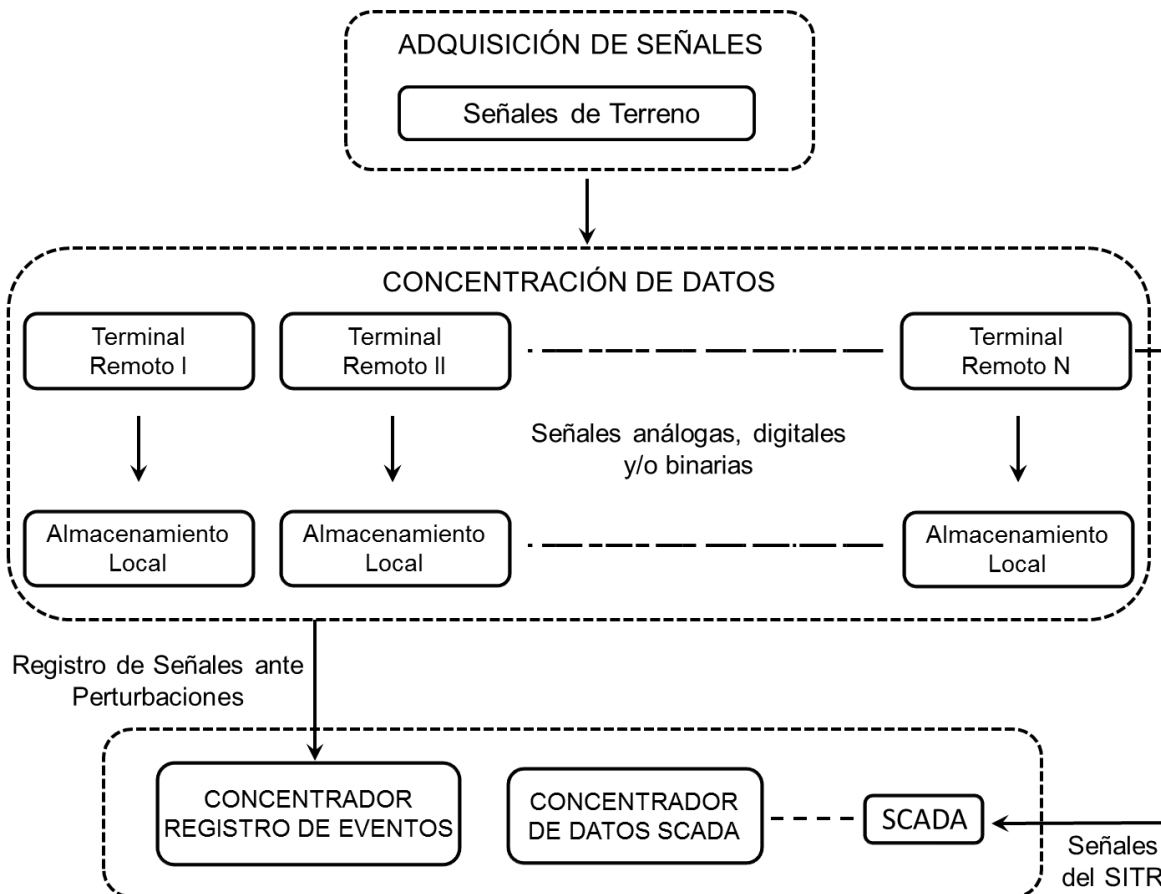
Figura 2: Arquitectura del módulo para registro de señales
