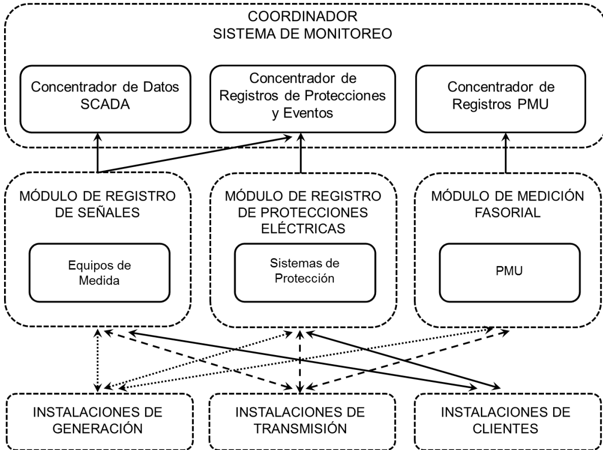
Figura 1: Arquitectura del Sistema de Monitoreo
