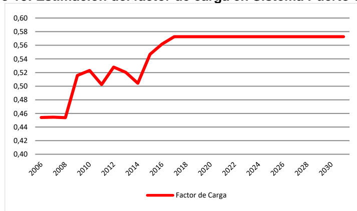
Gráfico 18: Estimación del factor de carga en Sistema Puerto Williams
