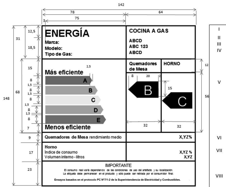
Figura 2: Dimensiones de etiquetado del artefacto para cocinar
